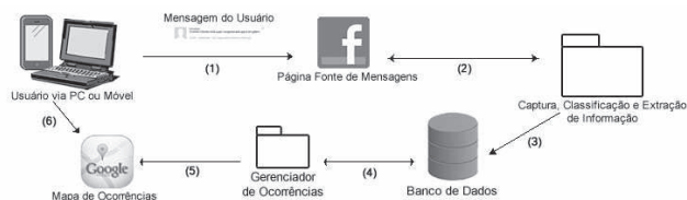
Figure 2. Diagrama de Funcionamento do Aplicativo EPITrans
